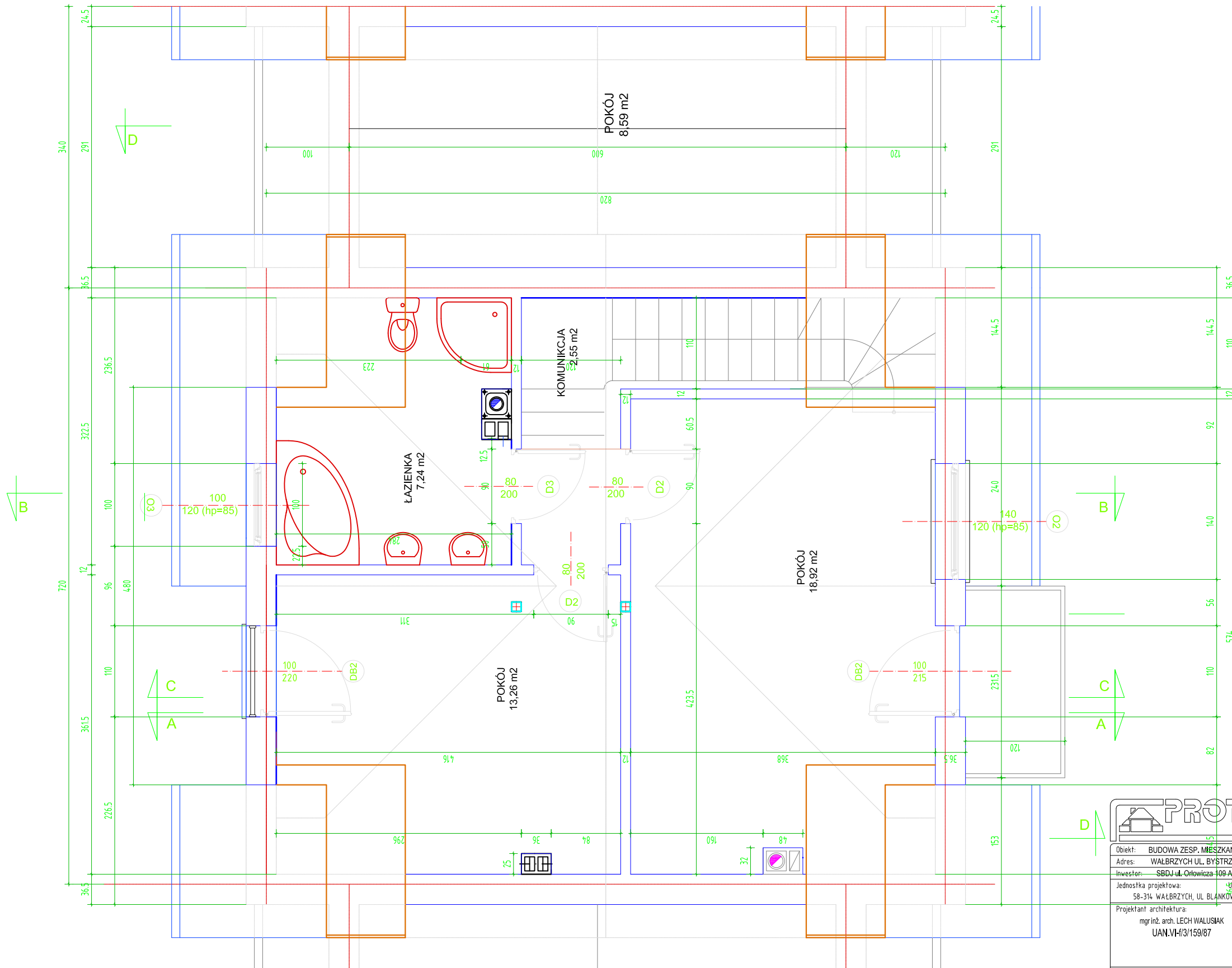
RZUT PODDZASZA 41,97 m 2 p.u.
